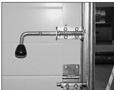
Рис. 41. Установка засова. Положение "открыто"
